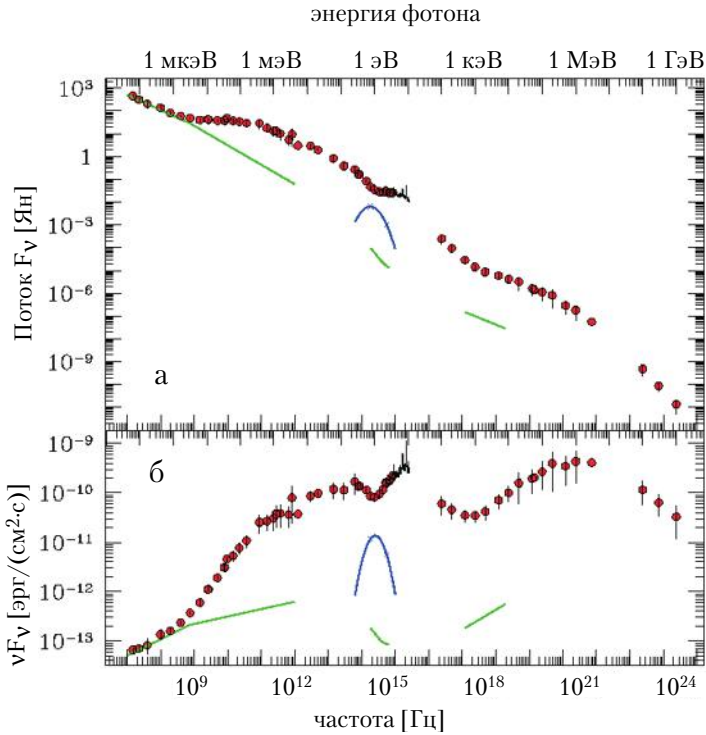
Рис. 2.5. Спектр квазара 3C273 от радио до \gamma -диапазона. Сверху – поток F_\nu в янских (единица измерения, 1 \text{ Ян} = 10^{-26} \text{ Вт}/(\text{м}^2 \cdot \text{Гц}) ). Снизу – величина \nu F_\nu , максимум которой указывает на частоты с максимальным энергосвещением.
