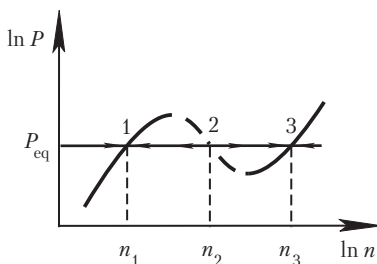
Рис. 4.2. К тепловой неустойчивости МЗС. Участок кривой P(n) с отрицательной производной соответствует неустойчивому состоянию.
