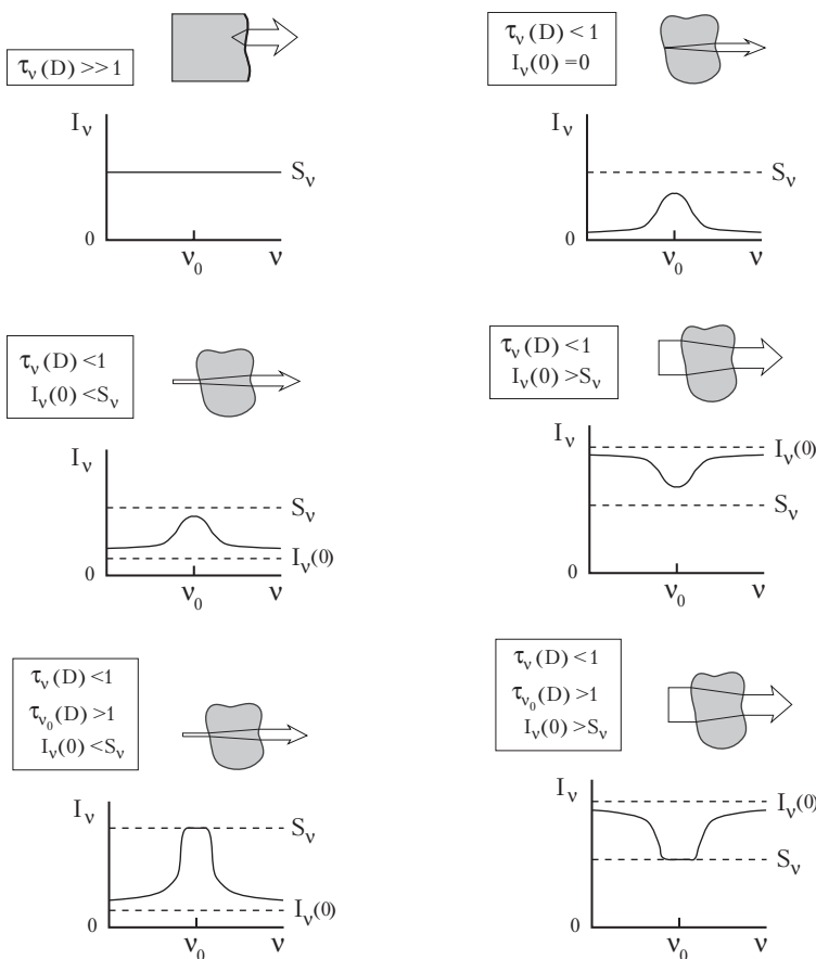
Рис. 2.4. Излучение спектральных линий в однородной среде. Если оптическая толщина излучающей области велика, линий нет (вверху слева). Оптически тонкая среда излучает эмиссионные линии, если подсветки сзади нет ( I(0) = 0 , справа вверху), или она слабая ( I(0) < S ). Линии поглощения появляются, если значение функции источника подсветки больше значения функции источника на данной частоте (справа внизу).
