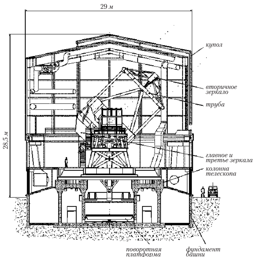
Рис. 3.5. Схематическое изображение одного из 4-х 8.2-м телескопов проекта VLT Южной Европейской Обсерватории на плато Паранал в чилийских Андах.
