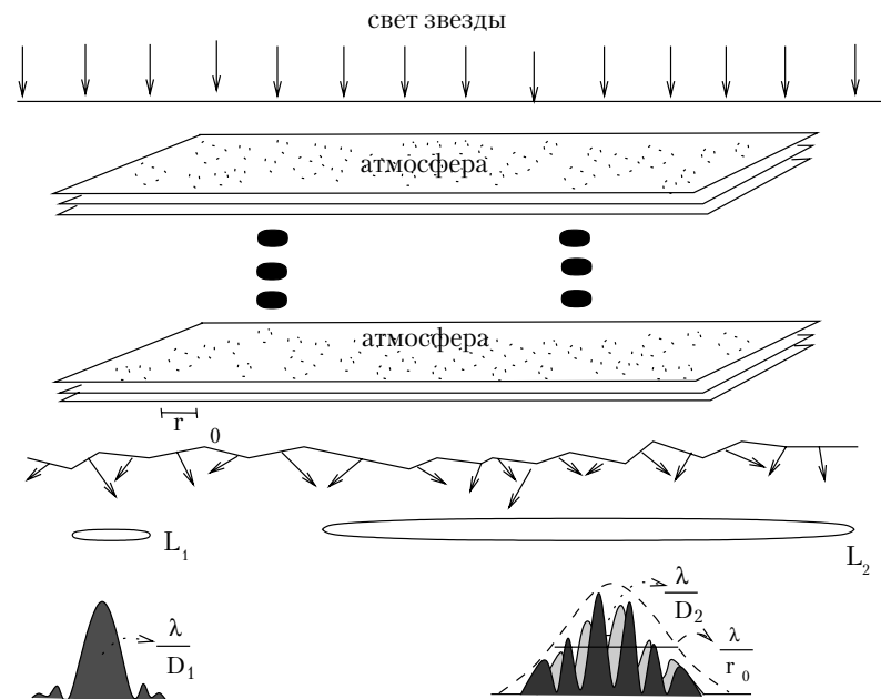
Рис. 3.7. Прохождение света через турбулентную атмосферу. Слева – регистрация телескопом малой апертуры D_1 , справа – телескопом большой апертуры D_2 \gg r_0 . r_0 – параметр Фрида, характеризующий масштаб турбулентности.
