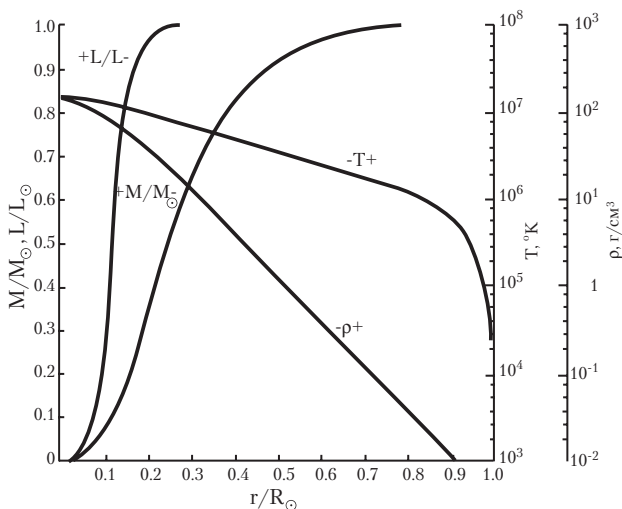
Рис. 5.4. Внутреннее строение Солнца в стандартной модели с химическим составом X=0.708 , Y=0.272 , Z=0.0020 , центральной плотностью \rho_c = 158 \text{ г см}^{-3} и центральной температурой T_c = 1.57 \cdot 10^7 \text{ К} . По данным из работы Guenther et al. ApJ v. 387 , p.372 (1992).
