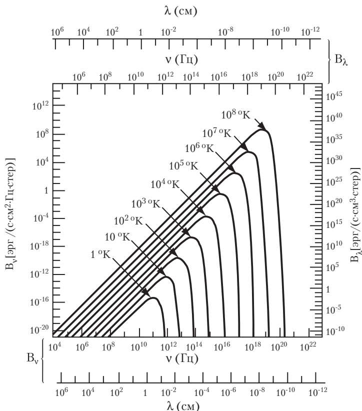
Рис. 2.3. Спектр АЧТ
