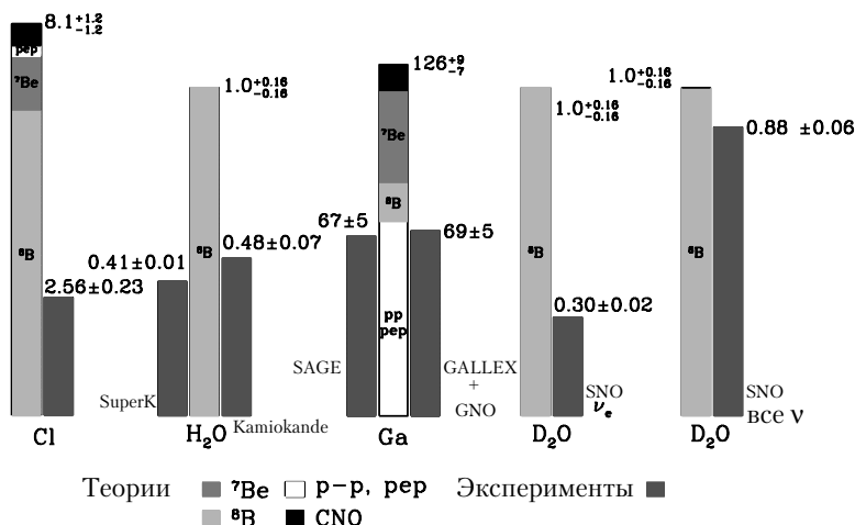
Рис. 5.3. Расчетные и экспериментально измеренные потоки солнечных нейтрино различными детекторами (в различных единицах для разных детекторов). Теория на уровне 5.3\sigma подтверждает эксперимент для всех сортов нейтрино, регистрируемых установкой SNO (последний столбец диаграммы).
