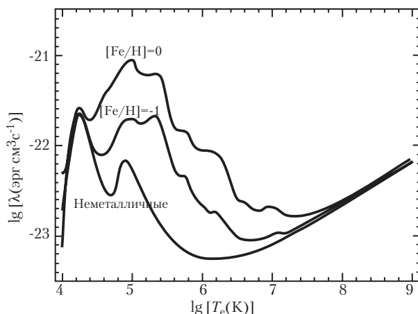
Рис. 4.1. Эффективность охлаждения разреженной космической плазмы \lambda(T) [эрг·см 3 /с] со столкновительным возбуждением и ионизацией. Приведены кривые для плазмы солнечного химического состава (верхняя кривая), с обедненным в 10 раз содержанием металлов (средняя кривая) и водородно-гелиевой плазмы (75% H, 25% He) без тяжелых элементов (нижняя кривая). Резкий скачок вблизи T \sim 10^4 К связан с ударным возбуждением второго (резонансного) уровня атомов водорода. На нижней кривой максимумы соответствуют водороду (слева) и гелию (справа). На верхних кривых появляются максимумы, соответствующие ударному возбуждению ионов углерода, кислорода, неона, кремния и железа. При T > 10^7 К эффективность охлаждения асимптотически стремится к зависимости \lambda(T) \propto \sqrt{T} , поскольку преобладает охлаждение тормозным излучением, зависящим от относительной (тепловой) скорости частиц.
