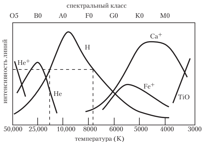
Рис. 5.5. Относительные интенсивности линий поглощения различных ионов в зависимости от эффективной температуры (спектрального класса звезды). Одной и той же интенсивности линий поглощения водорода может соответствовать разный спектральный класс (пунктир), поэтому для выбора спектрального класса нужно учитывать линии различных элементов.
