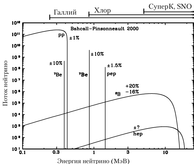
Рис. 5.2. Расчетный спектр потока солнечных нейтрино на Земле (в единицах [нейтрино/см 2 /с/МэВ]) в стандартной модели Солнца (J.Bahcall, M.Pinsonneault 2000) от различных реакций pp -цикла и эксперименты, способные регистрировать нейтрино различных энергий: Gallium – Ga-Ge эксперимент (SAGE: Лос-Аламосская Национальная Лаборатория, США и Баксанская нейтринная обсерватория, ИЯИ РАН, Россия; GALLEX: Гран-Сассо, Италия), Chlorine – Cl-Ar эксперимент (Хоумстейк, США), Super-K, SNO – черенковский эксперимент на воде H 2 O (Супер-Камиоканда, Япония) и на тяжелой воде D 2 O (Нейтринная обсерватория Садбюри, Канада). Процентами указана теоретическая неопределенность потока соответствующих нейтрино. См. подробнее на сайте J.Bahcall
