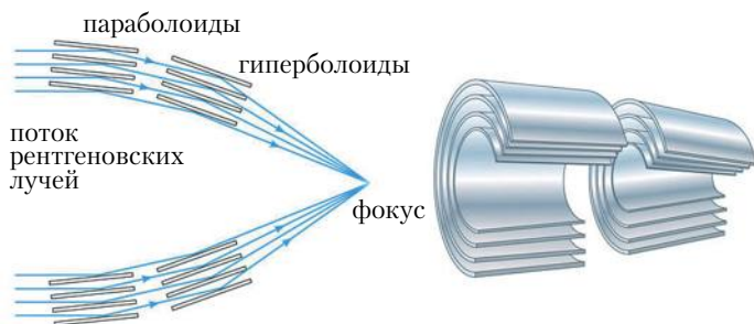
Рис. 3.6. Схема рентгеновского телескопа типа Уолтера с зеркалами косого падения.
