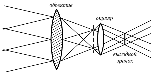
Рис. 3.4. К понятию выходного зрачка оптической системы.
