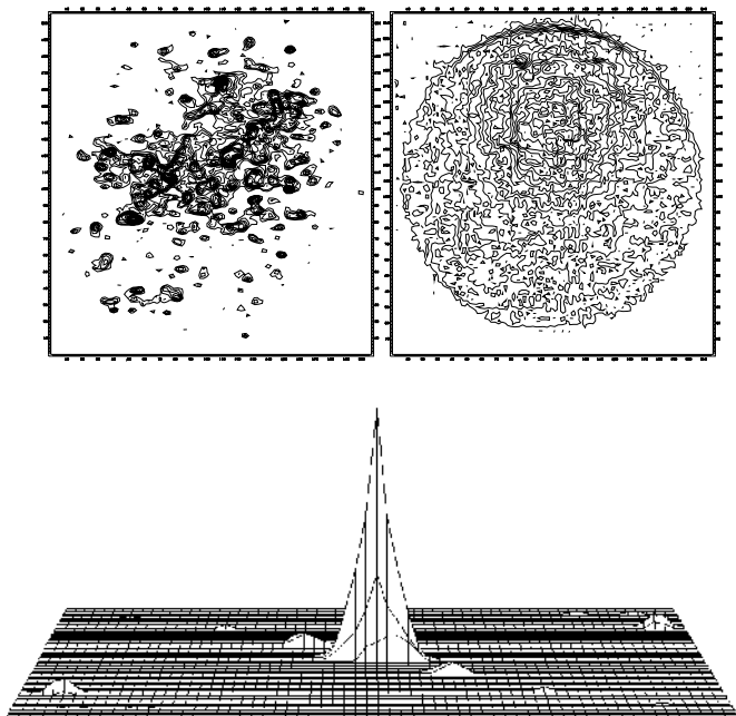
Рис. 3.8. Спеклограмма двойной звезды HR 4689 (вверху слева), сумма 128 спеклограмм (вверху справа) и автокорреляционная функция одной спеклограммы (внизу), на которой отчетливо видна двойственность источника.
