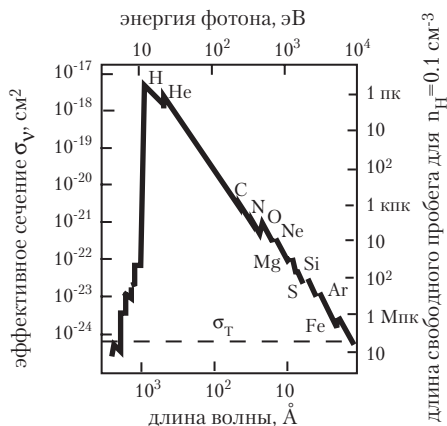
Рис. 3.3. Зависимость эффективного сечения поглощения атомов межзвездного газа со стандартным химическим составом от длины волны ионизирующего излучения (левая шкала). Правая шкала — длина свободного пробега квантов с данной энергией в межзвездной среде для концентрации межзвездного газа n_H = 0.1 частиц в \text{см}^3 при нормальном обилии гелия и более тяжелых элементов. Пунктиром показано томсоновское сечение рассеяния на свободных электронах, которое для фотонов с h\nu \ll m_e c^2 \approx 511 кэВ не зависит от энергии.
