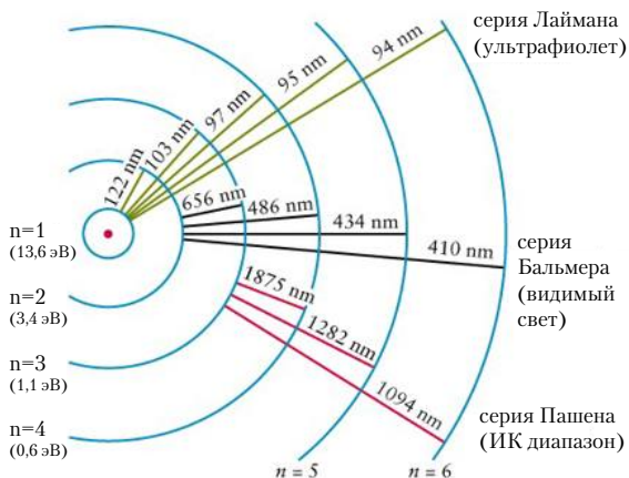
Рис. В.1. Основные спектральные серии водорода. Также показан потенциал ионизации с соответствующего уровня (в эВ).
