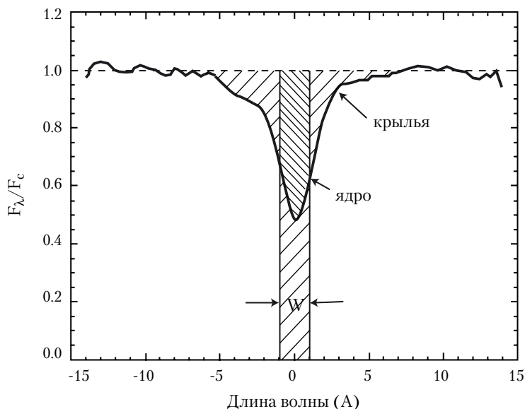
Рис. 5.6. Эквивалентная ширина спектральной линии. Поток в линии нормирован на поток в континууме.
