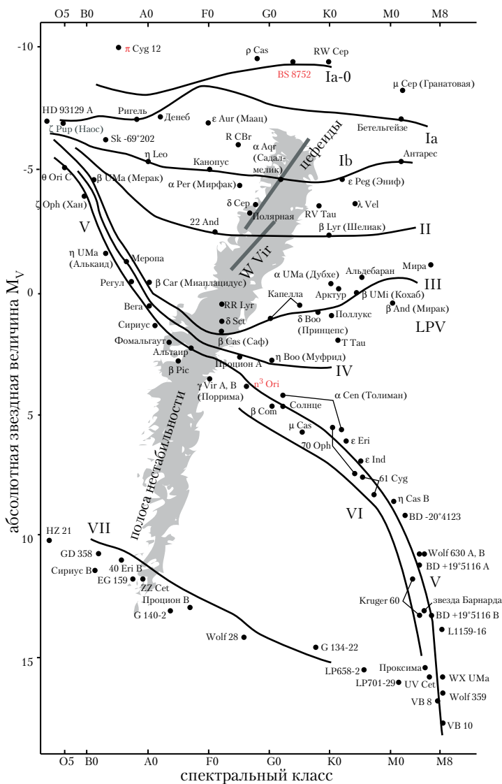
Рис. 5.1. Диаграмма Герцшпрунга–Ресселя для звезд в окрестности 25 пк от Солнца. Подробнее см. текст.
