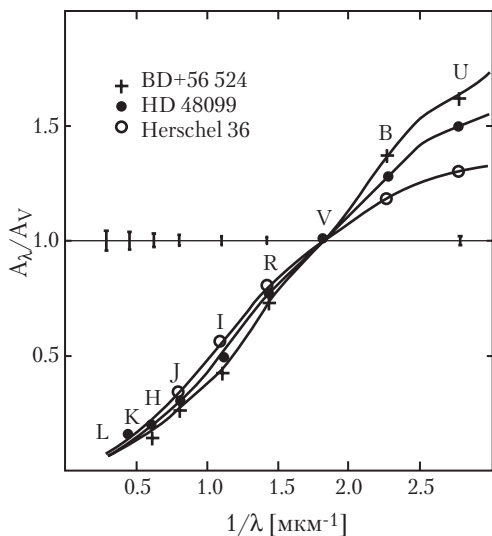
Рис. 3.2. Зависимость ослабления света (в зв. величинах) от обратной длины волны для различных направлений (на три различные звезды). Кривые нормированы на величину ослабления A = 1 в диапазоне V.
