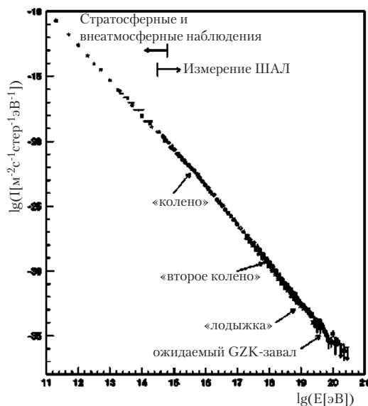
Рис. 4.3. Наблюдаемый энергетический спектр КЛ по данным различных экспериментов имеет степенной характер в диапазоне энергий от 10^{11} до 10^{20} эВ с небольшими изломами вблизи 10^{15.5} эВ («колено»), 10^{17.8} эВ («второе колено») и 10^{19} эВ («лодыжка»). Завал в спектре КЛ сверхвысоких энергий из-за взаимодействия с фотонами реликтового излучения (эффект Грайзена–Зацепина–Кузьмина) ожидается вблизи энергии 10^{19.6} эВ. Рисунок взят из обзора Nagano M., Watson A.A., Rev. Mod. Phys., 27 , p.689 (2000).
