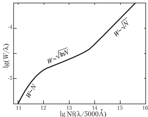
Рис. 5.7. Кривая роста для Солнца.
